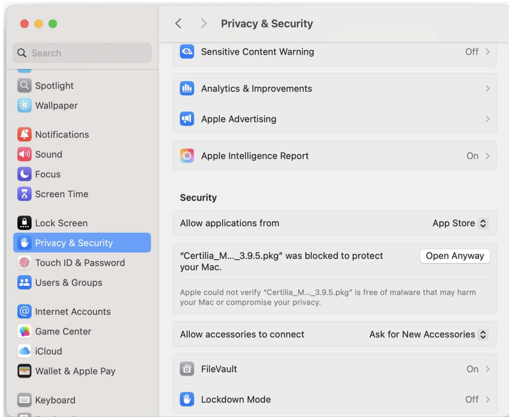
Slika 1.8 Pokretanje instalacije
