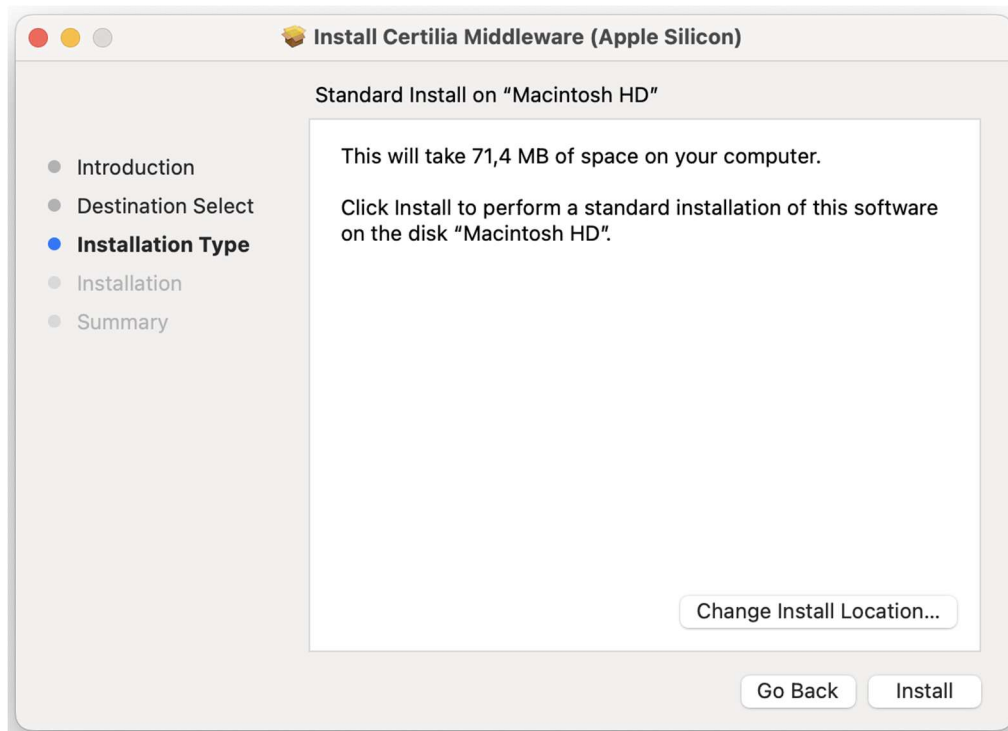
Slika 1.4 Dovršetak instalacije
