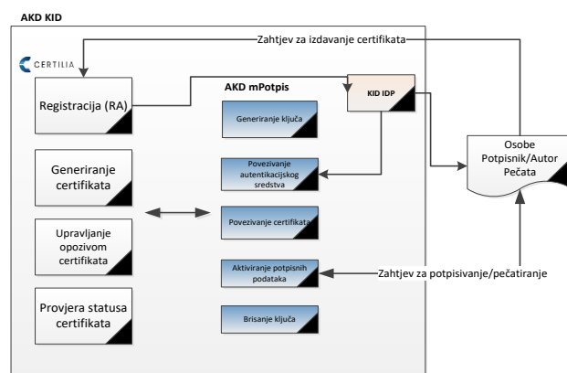
Slika 1a: CERTILIA mPotpis okruženje(SSASC)
